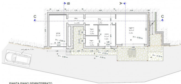
PIANTA PIANO SEMINTERRATO
